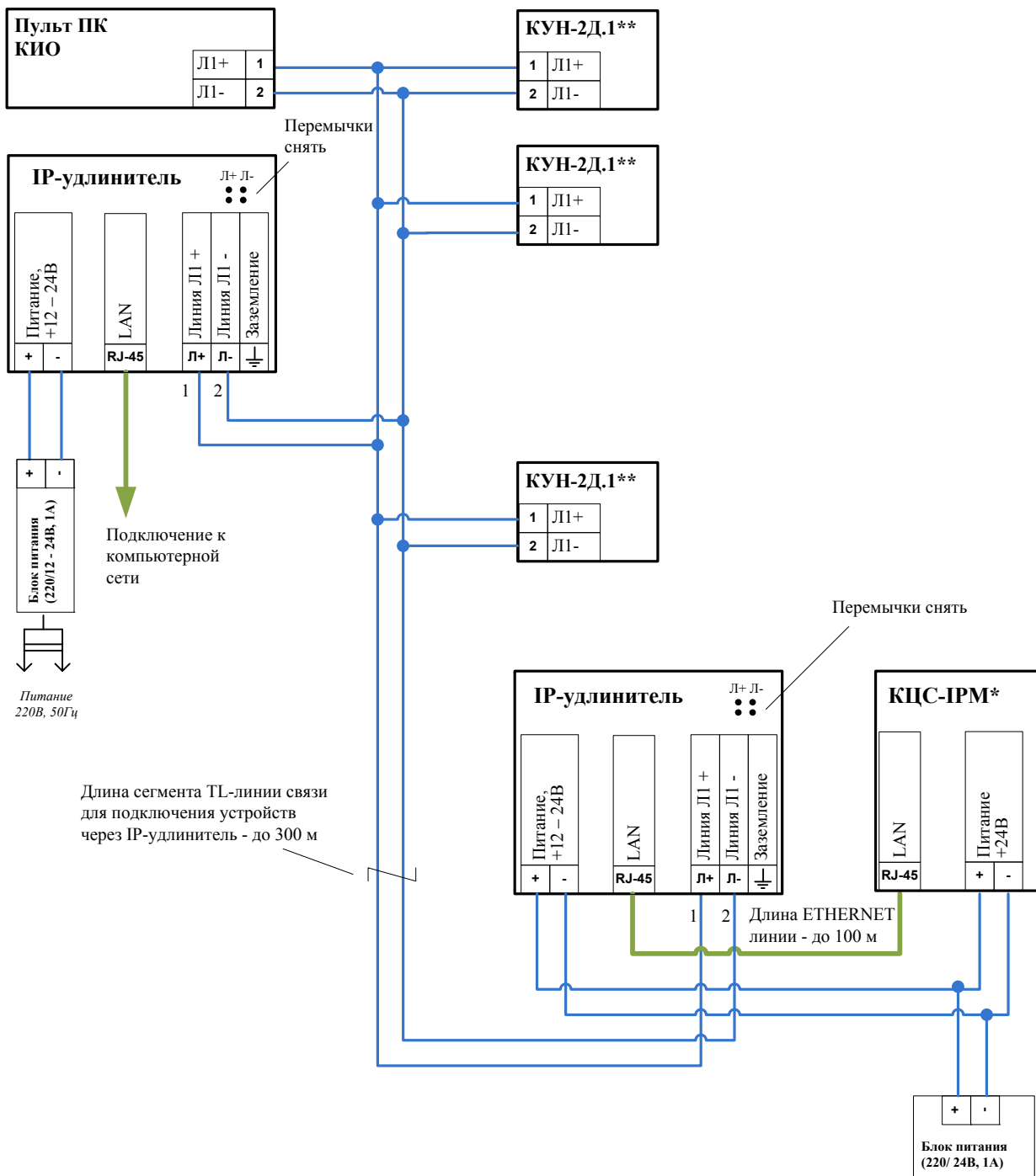
Рис. Б 3.11.7 Схема подключения КЦС-IPM* с использованием IP-удлинителя к TL-Линии связи.
