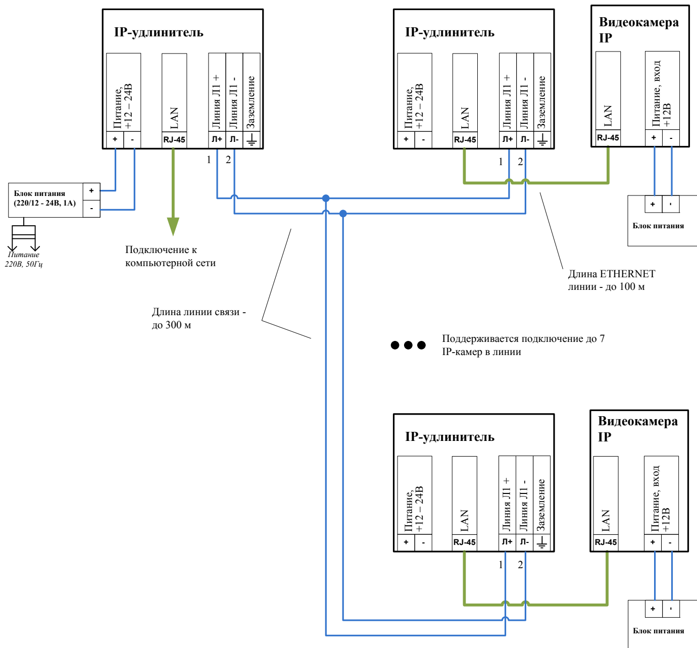
Рис. Б 3.11.5 Схема подключения IP-видеокамеры с использованием удлинителя – IP. Допускается подключать до 8 удлинителей – IP и 7 IP-видеокамер в одном сегменте
