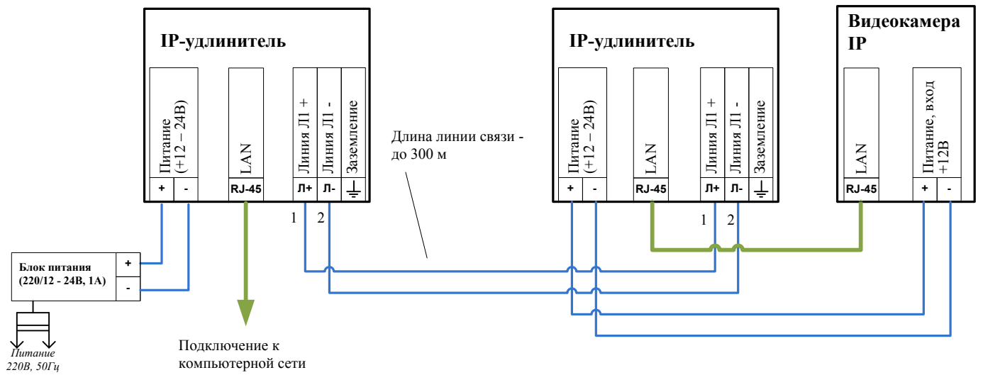
Рис. Б 3.11.4 Схема подключения IP-удлинителя с удаленной подачей питания на IP-камеру. Ограничение по току потребления камеры – до 1А.
