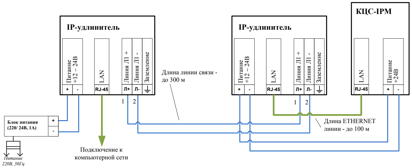
Рис. Б 3.11.3 Схема подключения IP-удлинителя с удаленной подачей питания на КЦС-IPM
