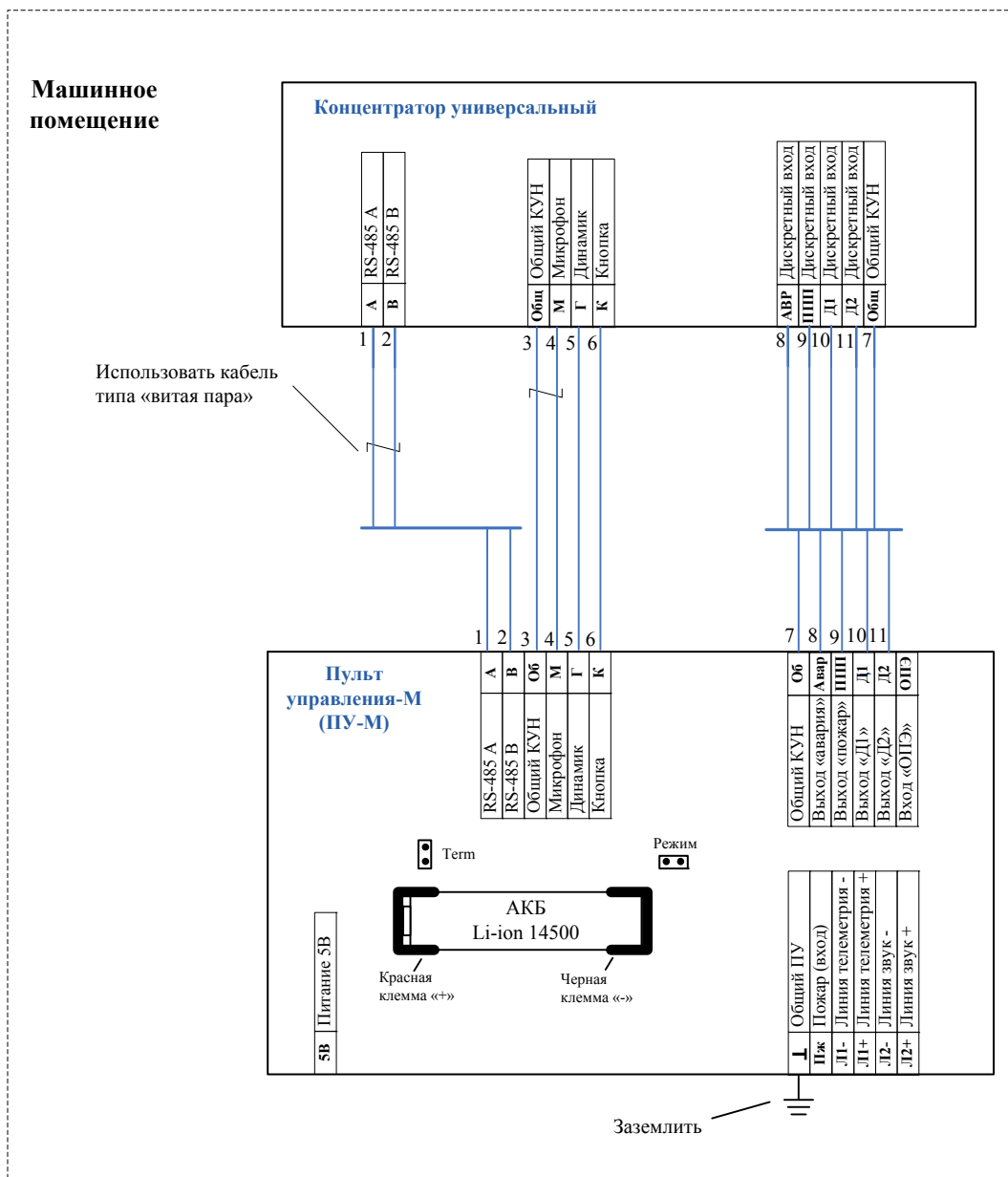
Рис. Б 2.20.6-2 Подключение Устройства переговорной связи лифта - М исполнение 2 (УПСЛ-М исп.2) к Концентратору универсальному (КУН) любого типа. Основные функции: связь лифта для пожарных, ремонтная связь лифта, связь с помещением для обслуживающего персонала.
