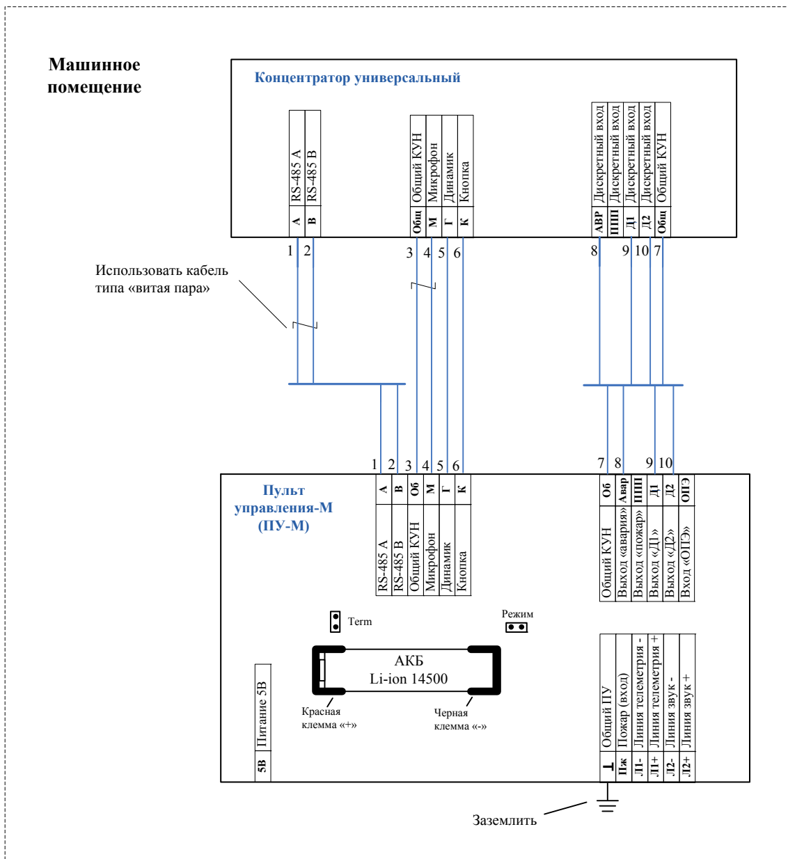
Рис. Б 2.20.5-2 Подключение Устройства переговорной связи лифта - М исполнение 1 (УПСЛ-М исп.1) к Концентратору универсальному (КУН) любого типа. Основные функции: ремонтная связь лифта, связь с помещением для обслуживающего персонала.
