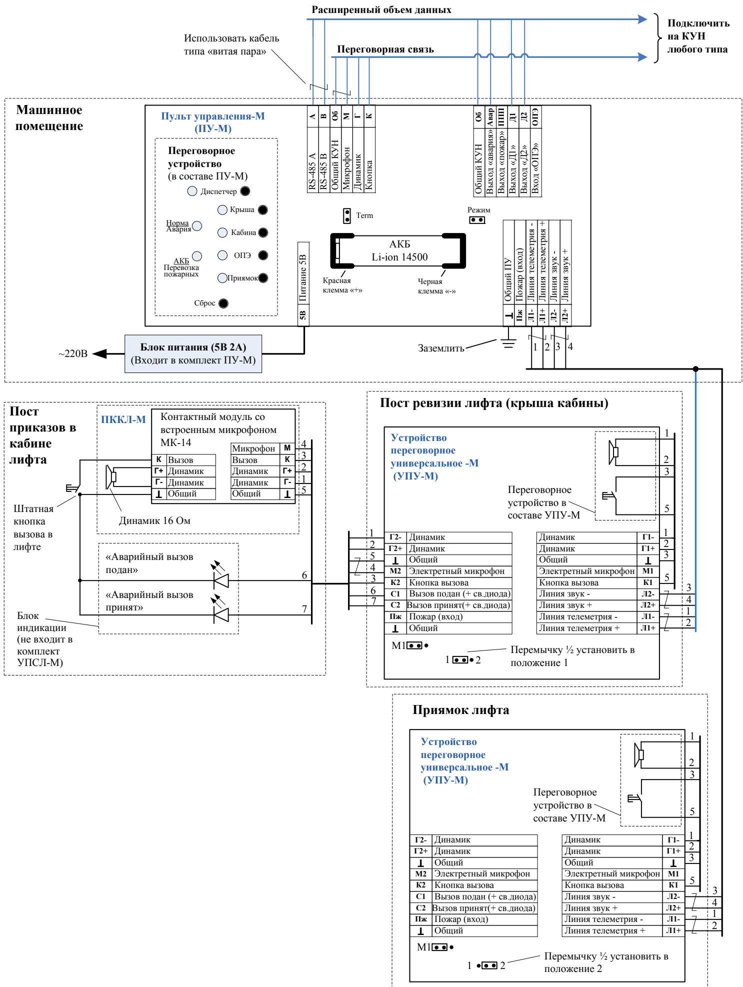
Рис. Б 2.20.3-2 Устройство переговорной связи лифта - М исполнение 1 (УПСЛ-М исп.1).
