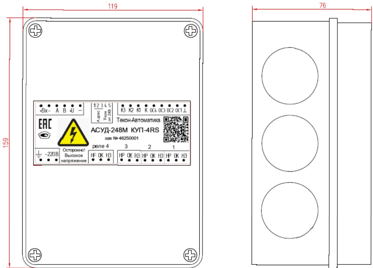
Рис.1. Корпус KVPI-4RS в исполнении IP54
