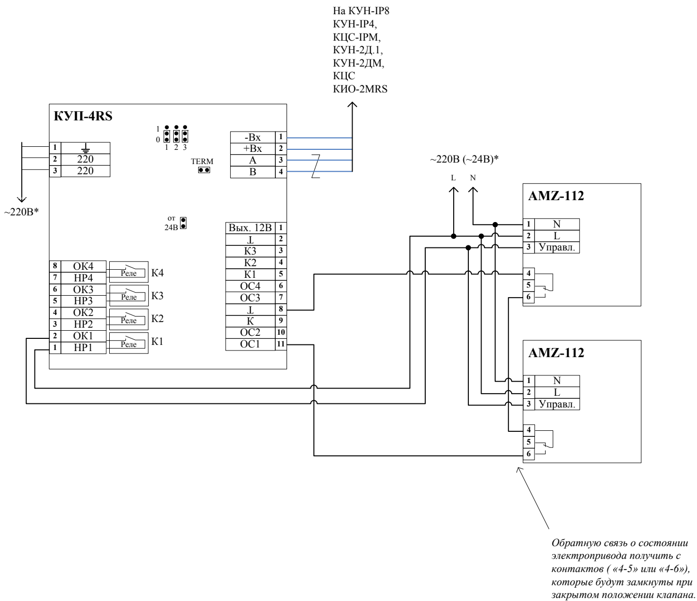
Рис. Б 4.7.1-2 Схема подключения концентратора управляющего-4RS (КУП-4RS) и электропривода AMZ-112.
