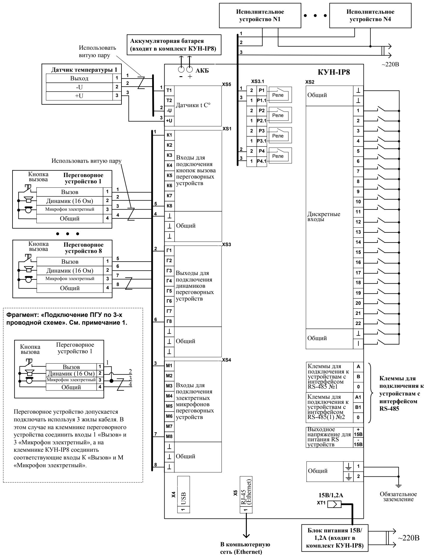
Рис. Б 2.3.1-3 Схема подключения концентратора универсального – IP8 (КУН-IP8).
