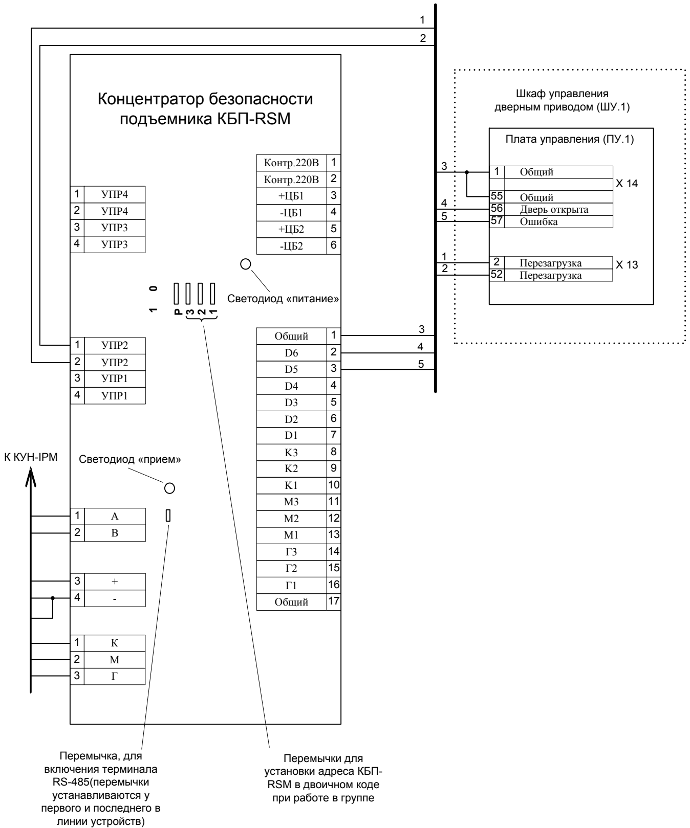
Рис. Б 4.5.1 Схема подключения концентратора безопасности подъемника КБП-RSM к приводу для двери серии DEMA-01-R-04-F, исполнение 1.
